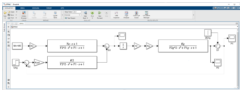
Рис. 4.5. Структурная схема САР ГПТ
