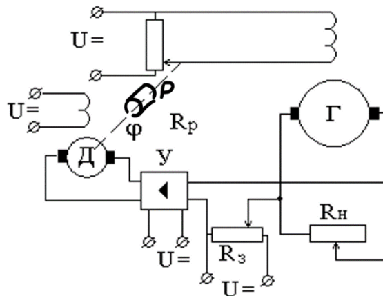
Рис. 4.1. Принципиальная схема САР ГПТ
